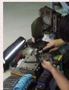
▲ハサミの切れ味調整作業、他にも機械の操作やメンテナンスをする担当作業もあります。
